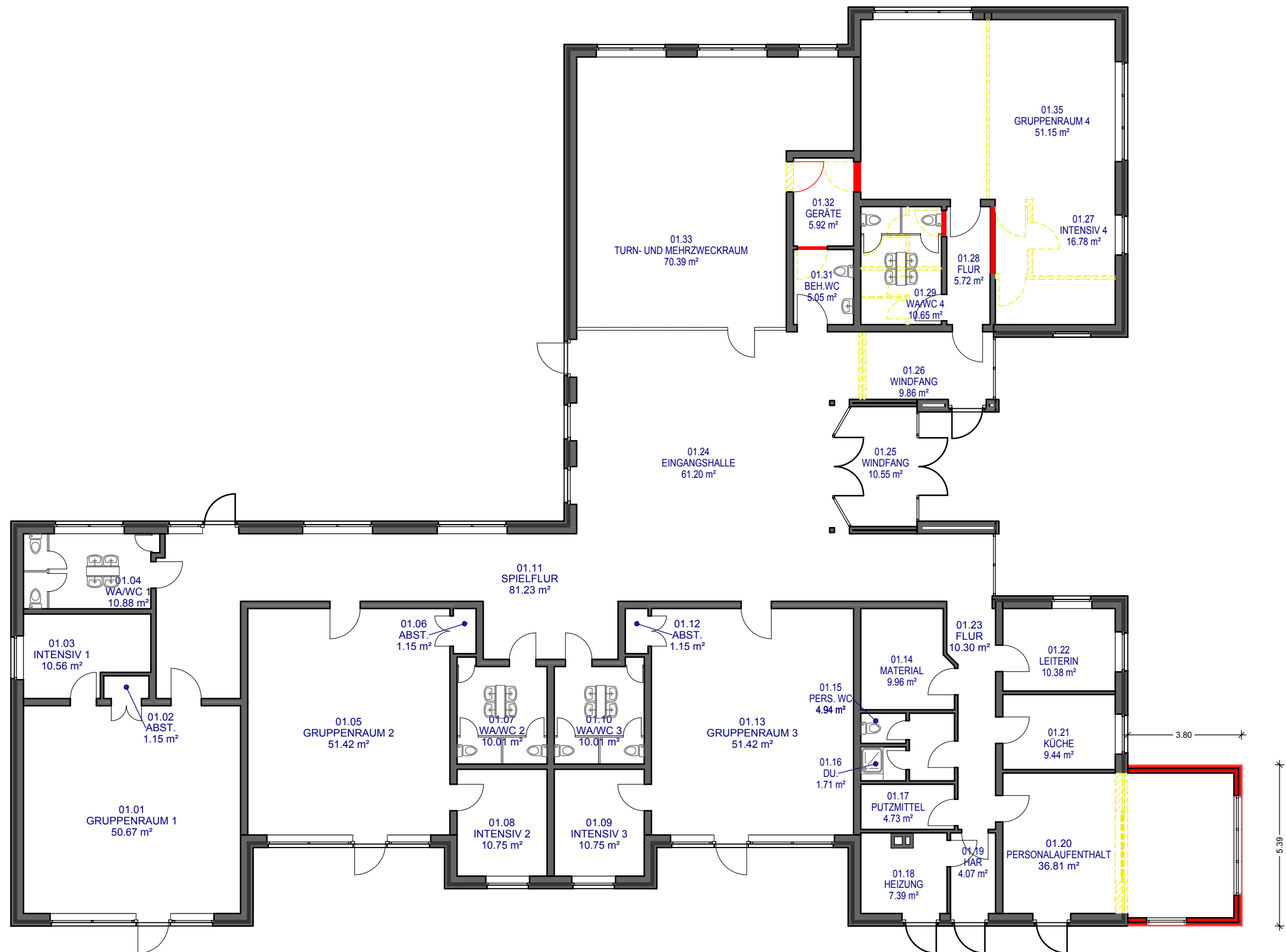
Kindergarten Osterscheps Grundriss
