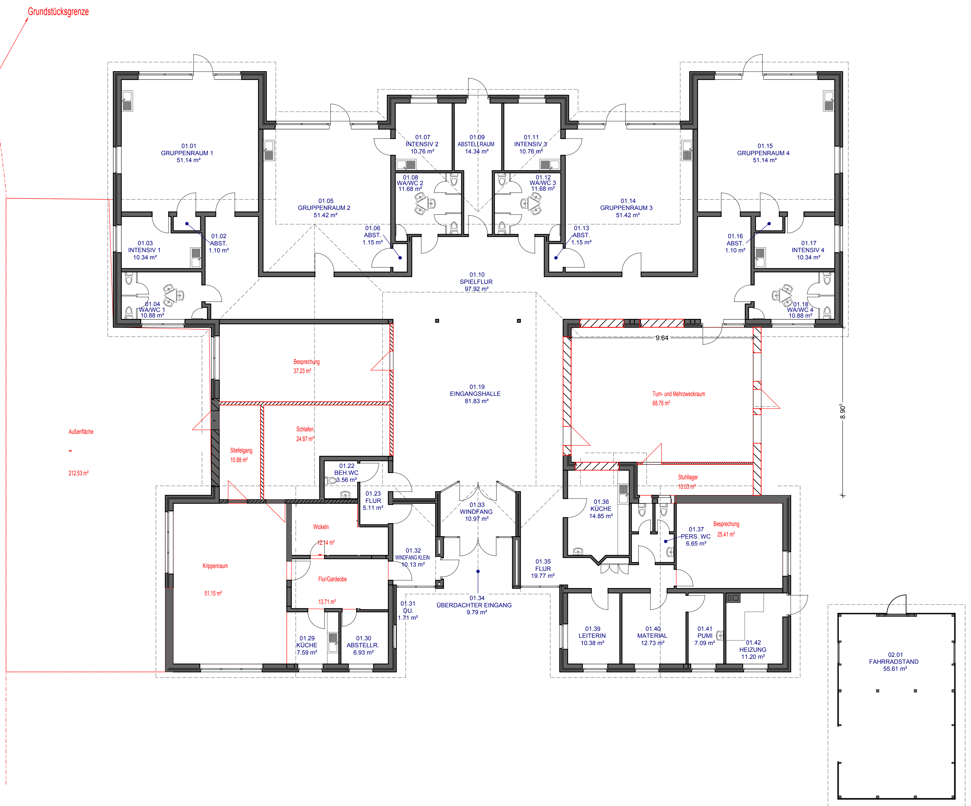
ÜBERSICHTSPLAN KINDERGARTEN JEDDELOH II GRUNDRISS (M.: 1:100)
